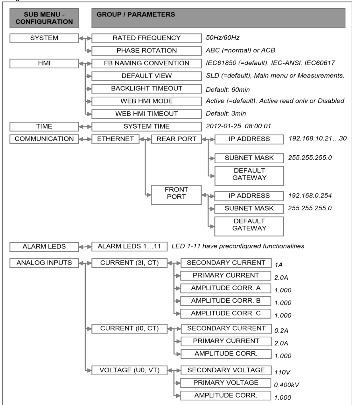
Fig. 10.11 The Configuration menu
