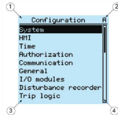
Fig. 12.5 Display layout
